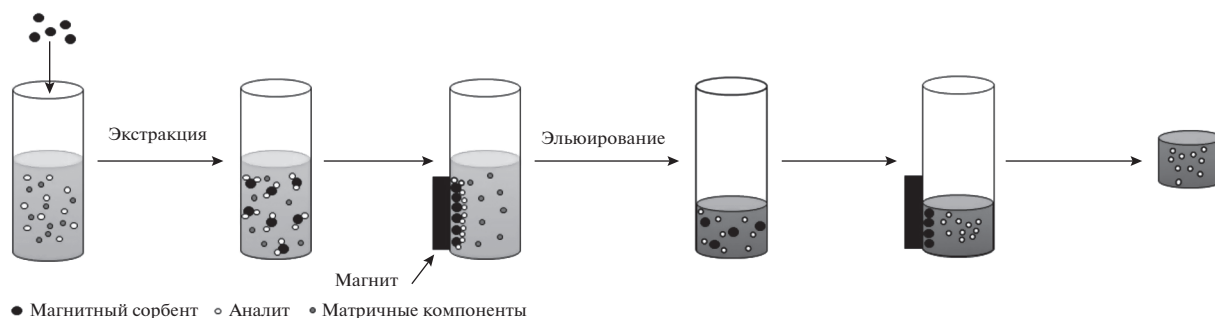
Рис. 3. Схема магнитной твердофазной экстракции.
